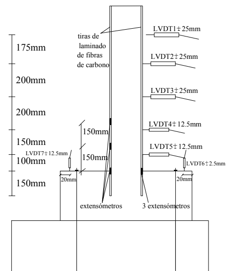
Figura 8: Transdutores de deslocamentos e extensômetros aplicados
