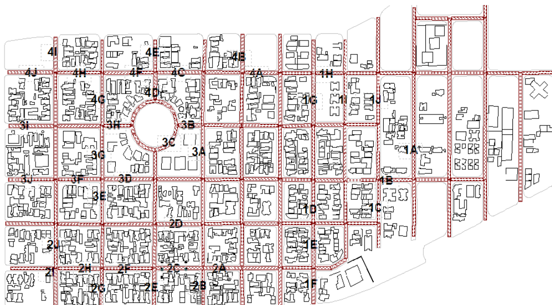
Figura 2 Localização dos pontos de contagem de tráfego e medição de ruído.
