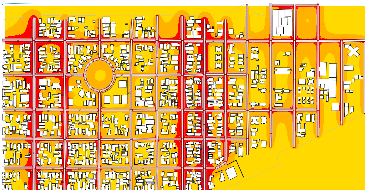
Figura 4 Mapa de ruído para o cenário existente
