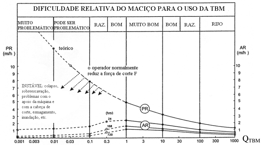
Figura 5 – Variação de PR e AR com o valor de Q_{TBM}
