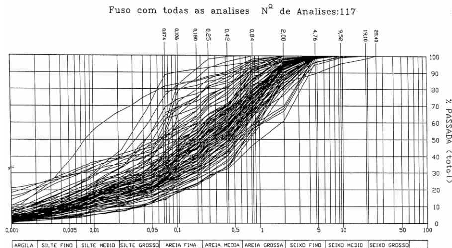
Fig.3.1 Fuso Granulométrico
