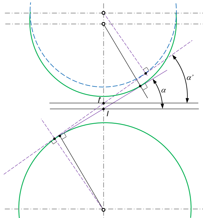
Fig. 77 Efeito da variação do entre-eixo no ângulo de pressão
