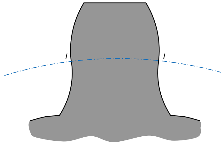
Fig. 67 Dente de perfil cicloidal
