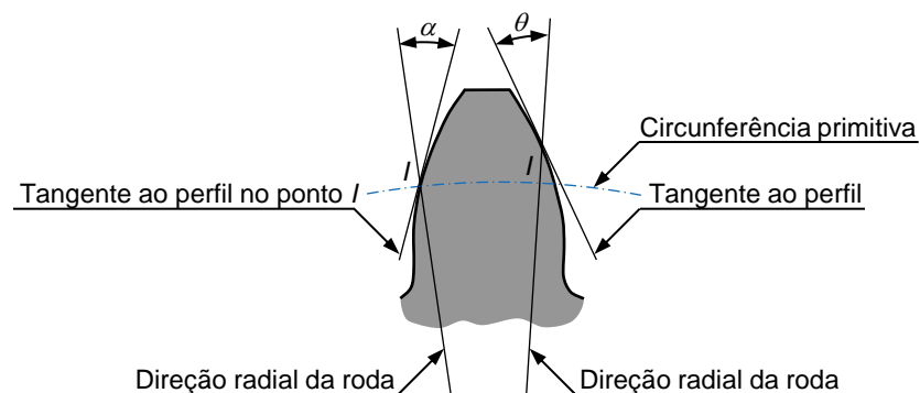
Fig. 59 Representação dos ângulos de incidência ( \theta ) e de pressão ( \alpha )
