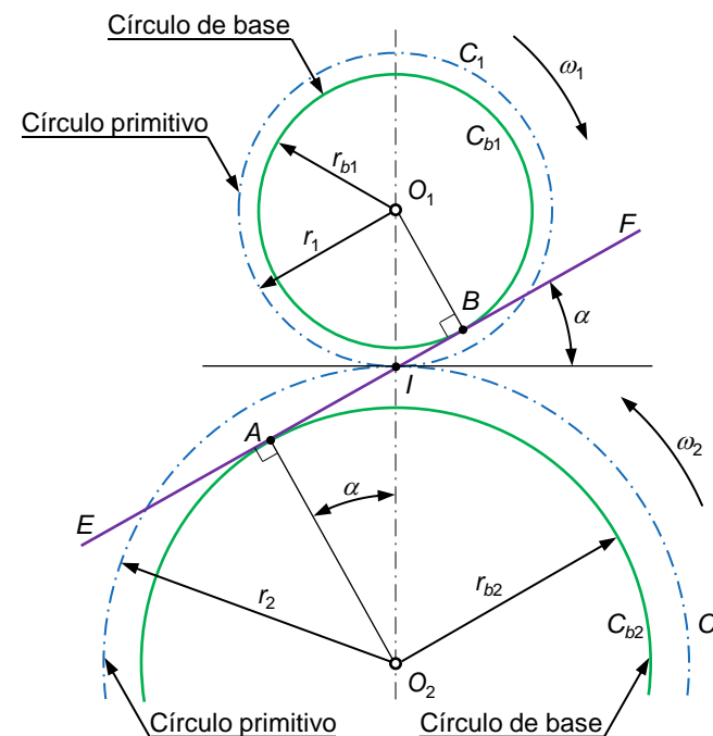
Fig. 72 Engrenamento de rodas dentadas e representação da linha de ação ou de engrenamento
