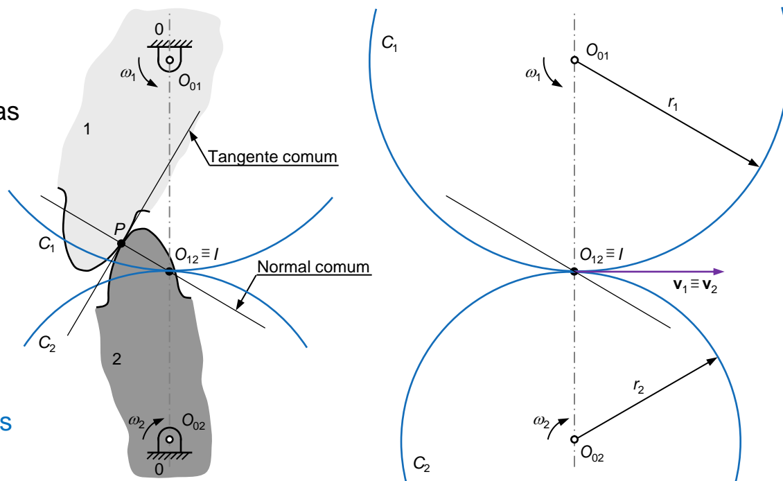
Fig. 79 Identificação das curvas primitivas numa engrenagem
