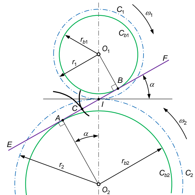
Fig. 75 Geração do perfil em evolvente
