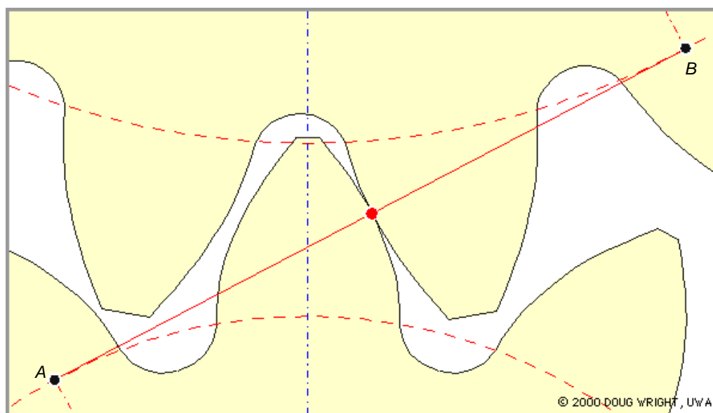
Fig. 72 Engrenamento de rodas dentadas e representação da linha de ação ou de engrenamento
