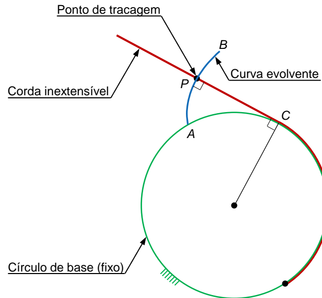
Fig. 68 Curva evolvente de círculo
