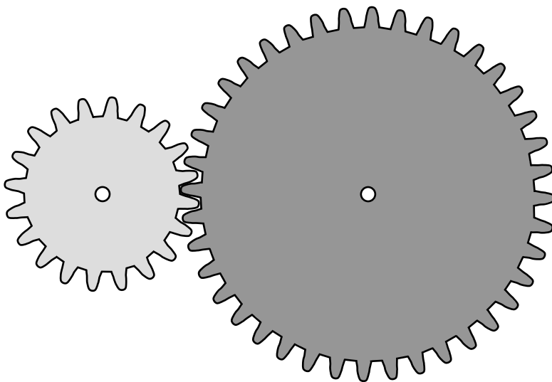
Fig. 61 Engrenagem com m_1=m_2=1 mm, z_1=20 e z_2=40
