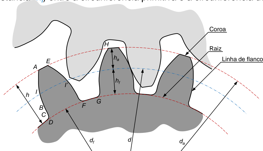
Fig. 56 Nomenclatura fundamental de uma engrenagem cilíndrica de dentes retos
