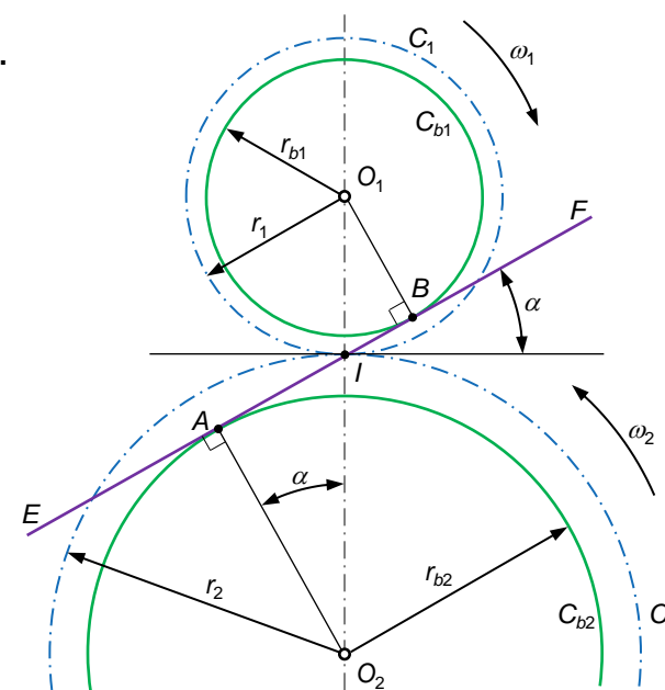
Fig. 74 Linha de ação ou de engrenamento
