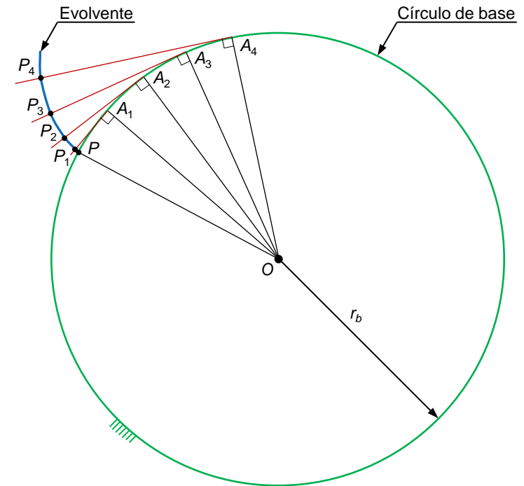
Fig. 70 Traçado de uma curva evolvente de círculo
