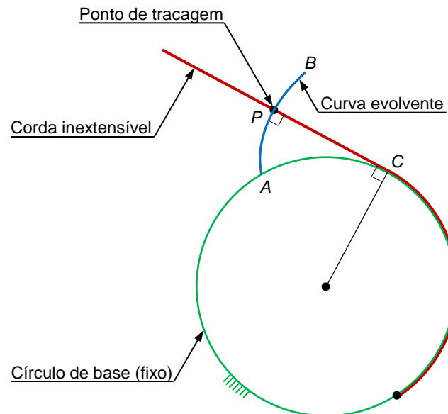
Fig. 69 Curva evolvente de círculo
