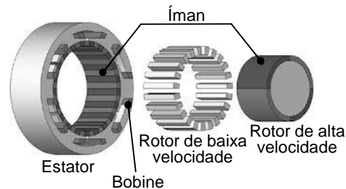
Fig. 48 Esquema de uma engrenagem magnética
