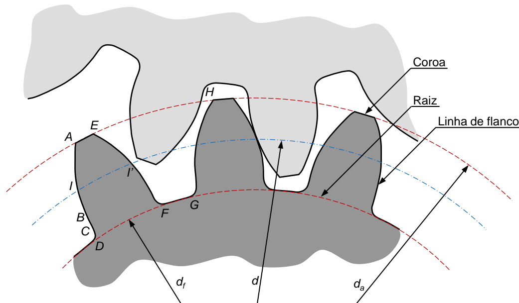
Fig. 53 Nomenclatura fundamental de uma engrenagem cilíndrica de dentes retos
