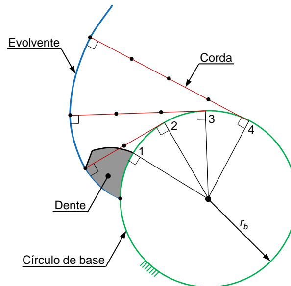
Fig. 71 Dente gerado em evolvente de círculo
