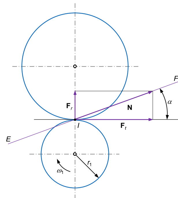
Fig. 78 Forças de engrenamento
