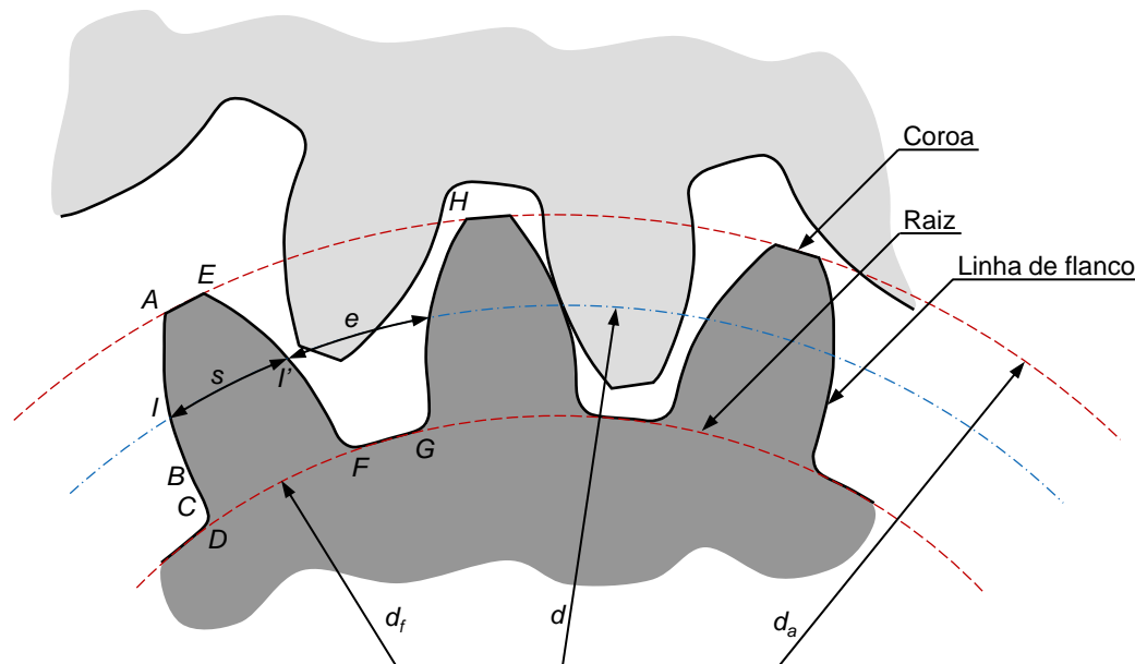
Fig. 58 Nomenclatura fundamental de uma engrenagem cilíndrica de dentes retos
