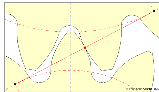
Fig. 5 Engrenamento de rodas conjugadas
