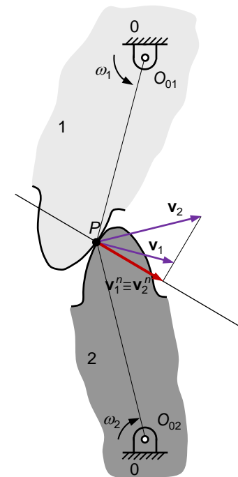
Fig. 81 Velocidades do ponto de contacto
