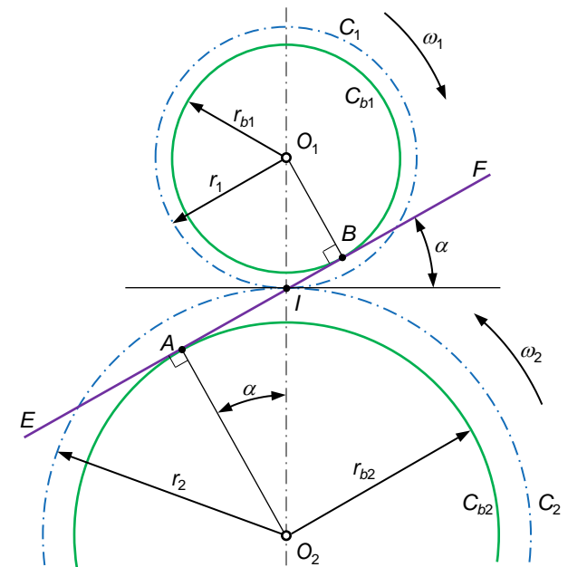
Fig. 73 Linha de ação ou de engrenamento
