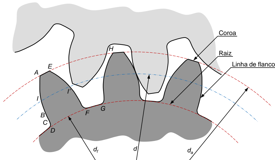
Fig. 52 Nomenclatura fundamental de uma engrenagem cilíndrica de dentes retos
