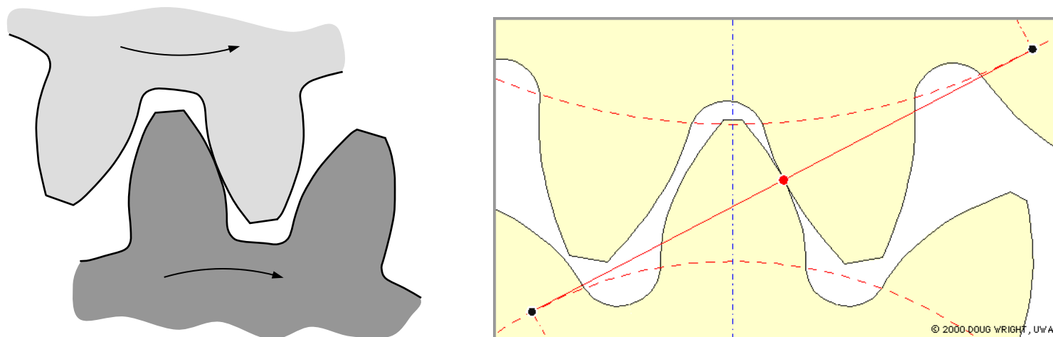
Fig. 63 Setores de duas rodas dentadas com perfis conjugados e engrenamento de rodas conjugadas
