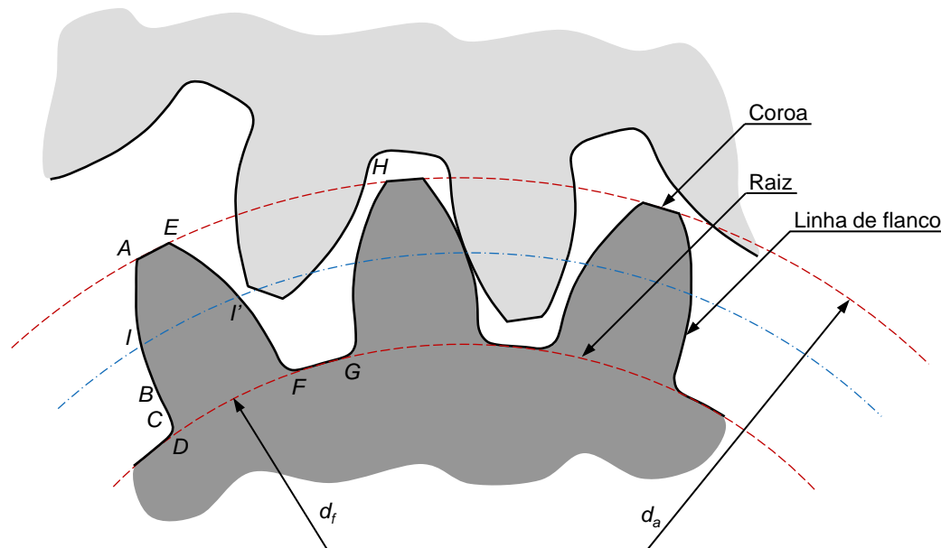
Fig. 51 Nomenclatura fundamental de uma engrenagem cilíndrica de dentes retos
