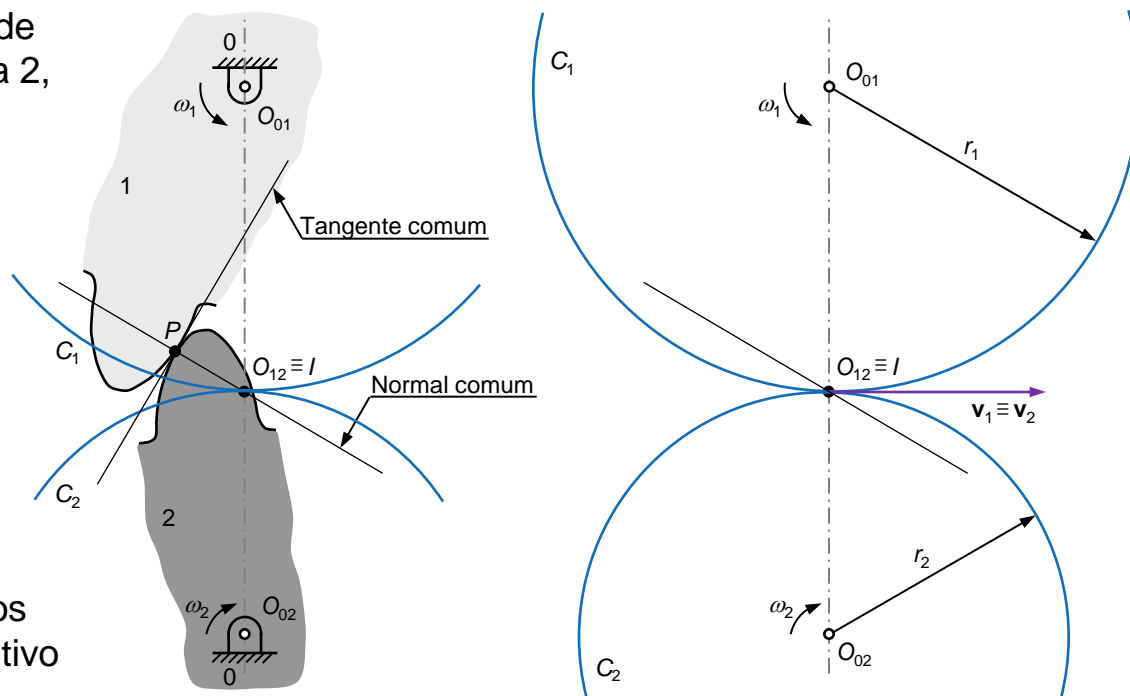
Fig. 80 Velocidade do ponto primitivo
