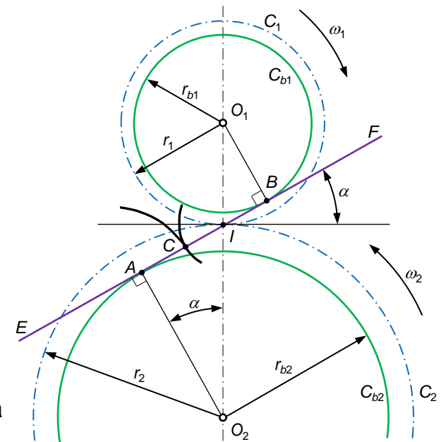
Fig. 76 Geração do perfil em evolvente
