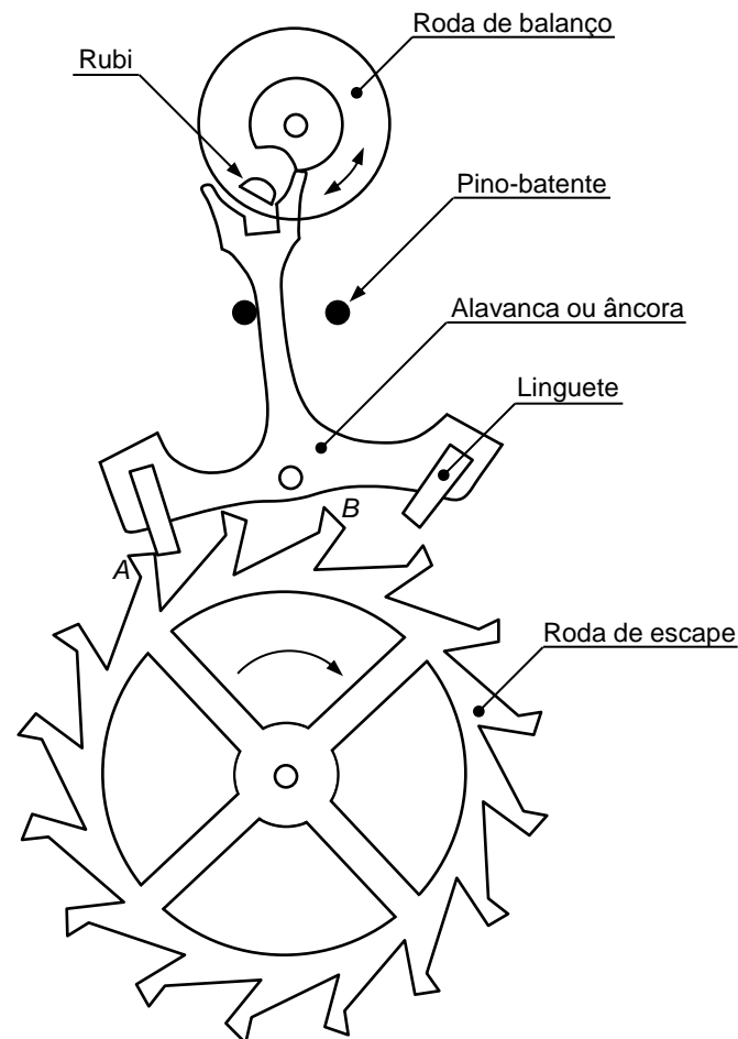
Fig. 49 Roda de balanço usada em relógios
