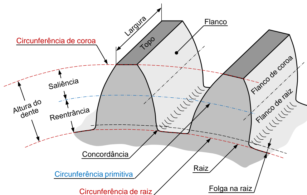
Fig. 50 Setor de uma roda cilíndrica exterior de dentes retos
