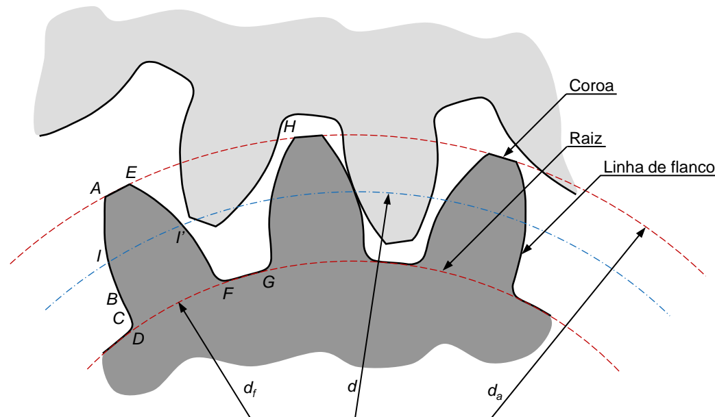
Fig. 54 Nomenclatura fundamental de uma engrenagem cilíndrica de dentes retos
