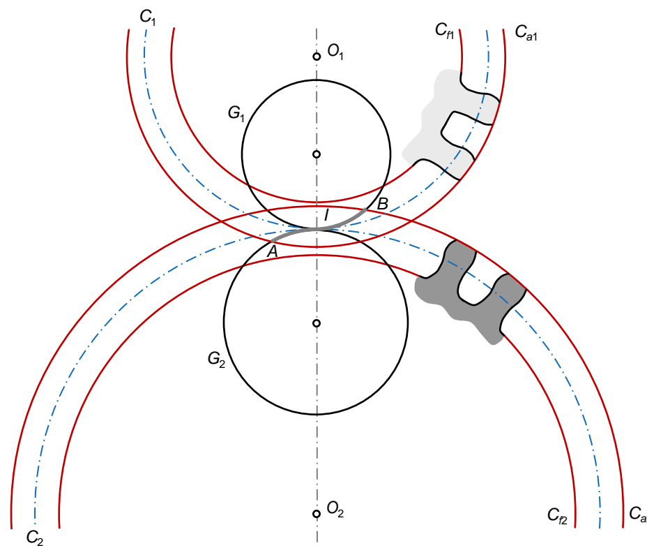
Fig. 66 Linha de ação numa engrenagem de dentado reto de perfil cicloidal
