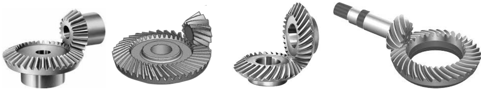
Fig. 41 Engrenagens cónicas de dentes retos, helicoidais, espirais, hipoide
