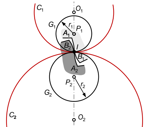
Fig. 65 Dentado cicloidal
