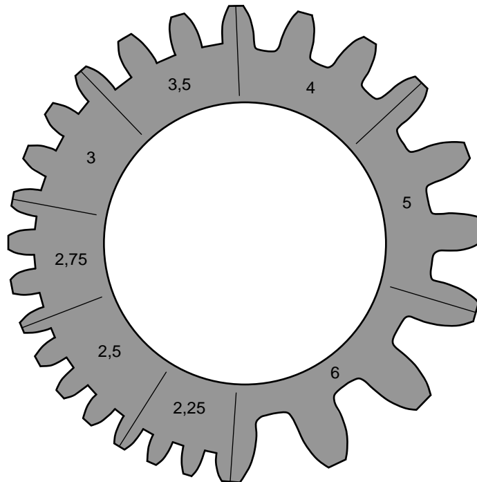
Fig. 60 Relação entre o módulo, tamanho dos dentes e número de dentes
