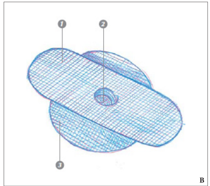
FIGURA 9. Método de Gilbert – Prolene Hernia System (PHS). A: Prótese de polipropileno de duas camadas (1 e 3) unidas por um conector (2). B: Aplicação da prótese (em: Hernia inguinocrural 1 )
