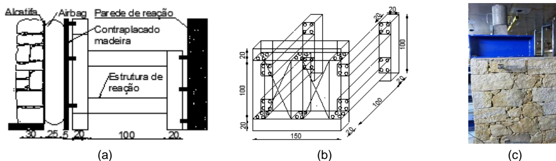
Fig. 4 – Configuração do ensaio para fora do plano (dimensões em cm): (a) esquema do ensaio em perfil; (b) estrutura com perfis metálicos HEB200; (c) aplicação da carga vertical nas paredes transversais
