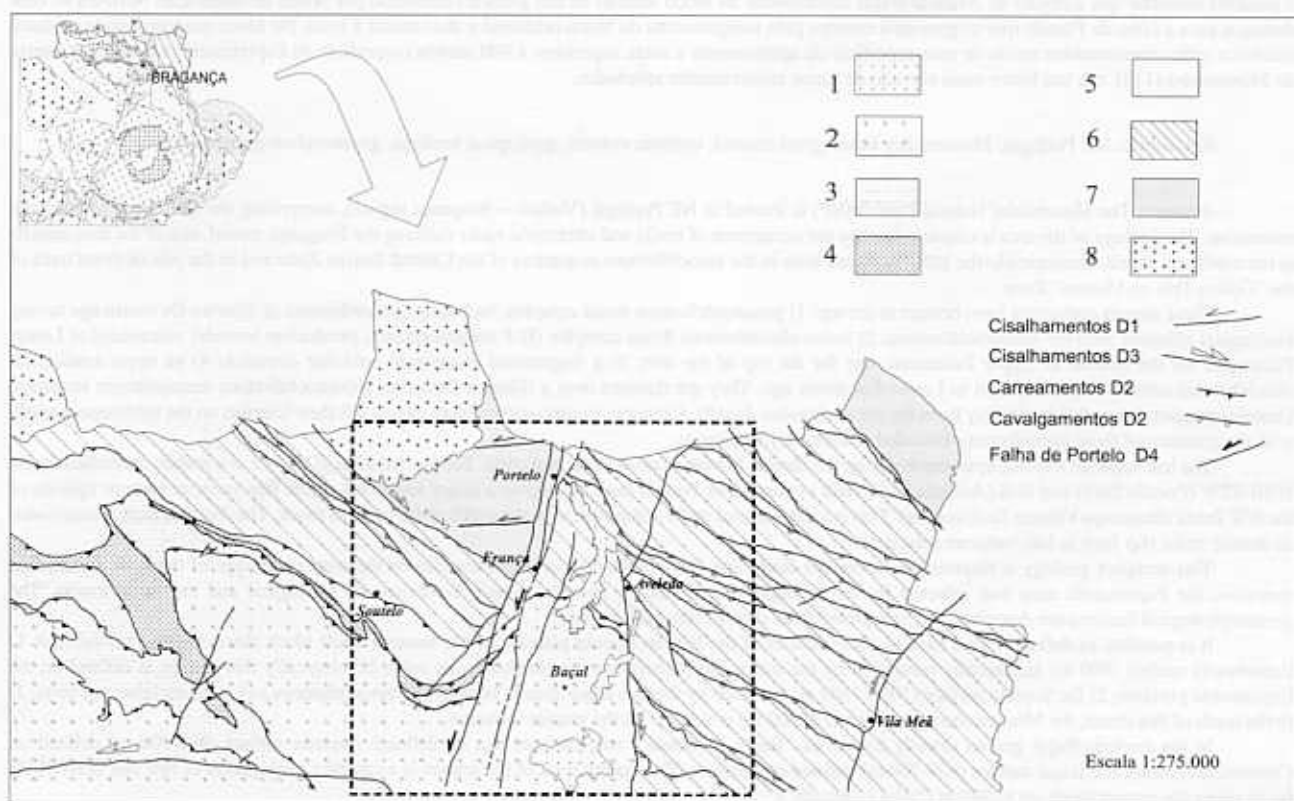
Fig. 1 – Enquadramento geológico da área estudada na geologia do Nordeste transmontano (adaptado de MEIRELES et al. , 1995). Legenda: 1 – Depósitos Terciários; 2 – Complexo Alóctone Superior; 3 – Complexo Alóctone Intermediário; 4 – Complexo Alóctone Inferior; 5 – Parautoctone; 6 – Subautoctone; 7 – Autoctone; 8 – Rochas Graníticas.
