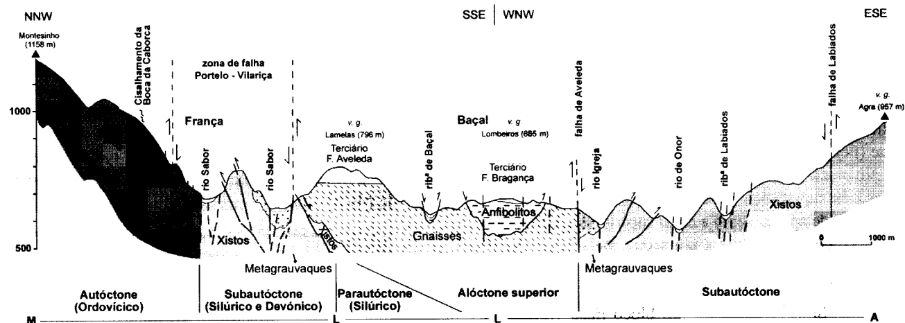
Fig. 3 – Perfil geológico esquemático segundo os vértices geodésicos Montesinho/Lamelas/Lombeiro/Agra (MLLA). É realçado o graben da Baixa Lombada definido pelo abatimento do bloco leste do acidente tectónico Bragança-Vilarica.
