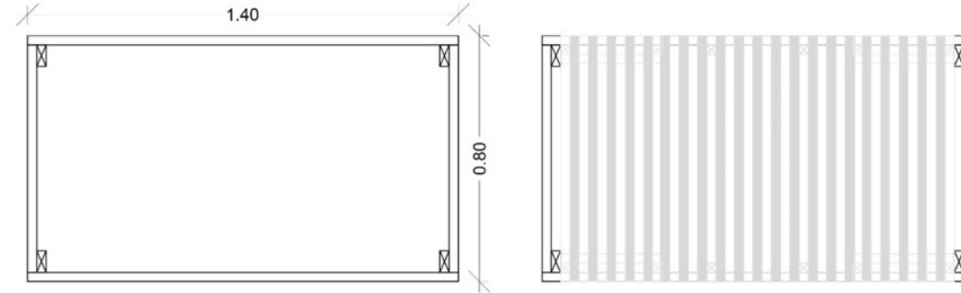
Planta | O Módulo da Box + Mesa + Banco
