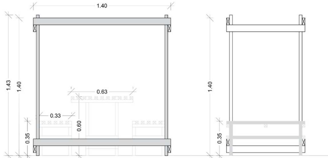
Corte | O Módulo da Box + Mesa + Banco
