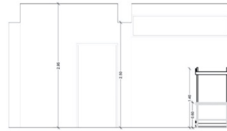
Corte A
