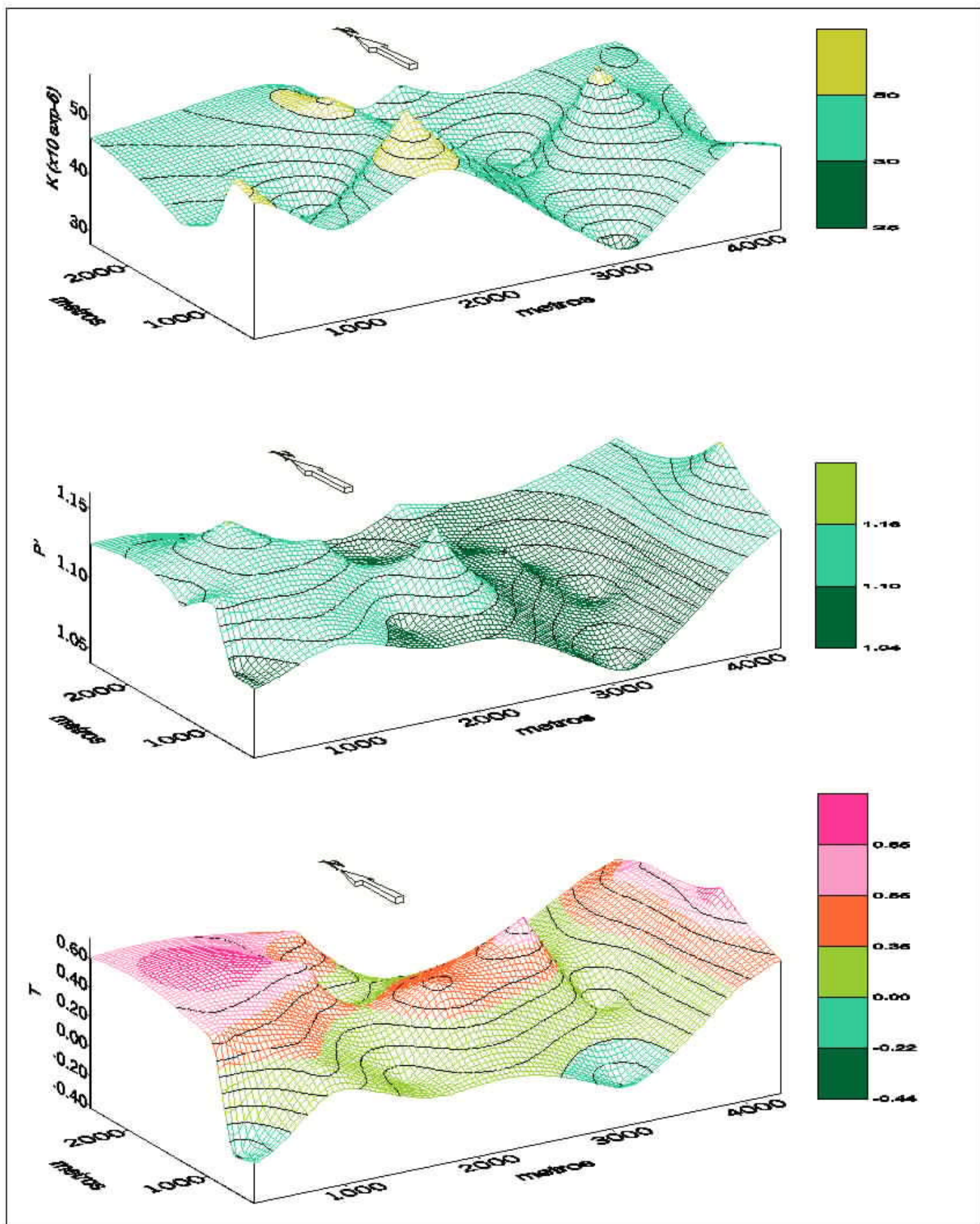
Figura.IV.48- Representação da variação de K, de P' e de T no maciço granítico de Caminha.
