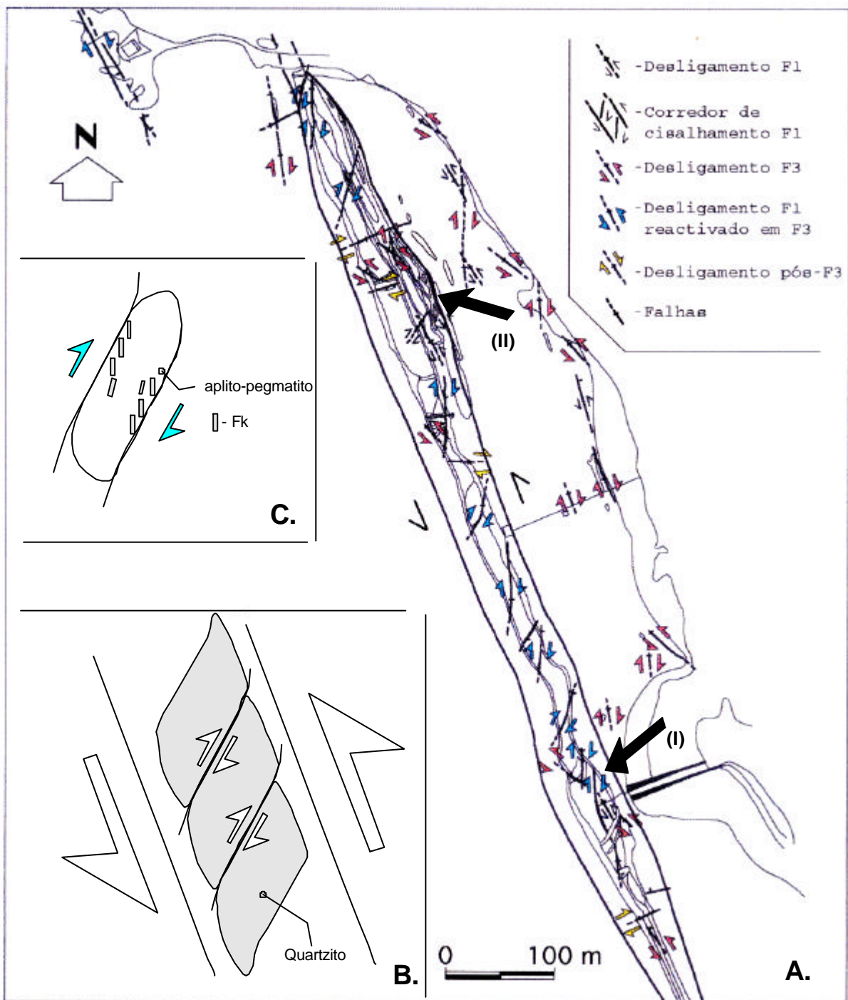
Figura.IV.14-A.Cartadecisalhamentos,deumsectorestudado(PraiaNorte-VianadoCastelo),evidenciando umcorredordecisalhamentocomestruturadominó.B.Representaçãoesquemáticadaestruturadominó horizontaledaformasigmoidaldoquartzito.C.Reactivaçãodecisalhamentos F_1 em F_3 (I)e(II)Localização dossectoresaondeseefectuaramos estudos dedeformação finita a 2D.
