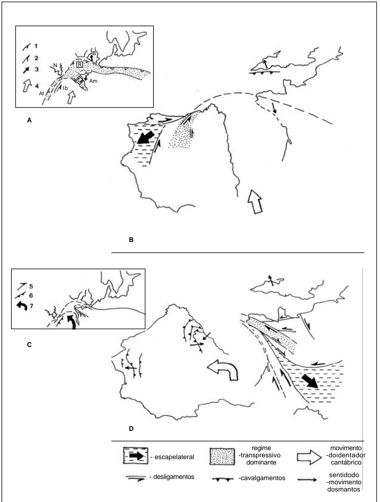
Figura II.11-Modelo de evolução geodinâmica do Arco Ibero-Armoricano. Devónico Superior: A- modelo de placas tectónicas; B-esquema de geodinâmica do Arco Ibero-Armoricano. Carbónico Médio/Superior: C-modelo de placas tectónicas; D-esquema de geodinâmica do Arco Ibero-Armoricano. Adaptado de Ribeiro & Dias (1995). Am-Armórica; Ib-Ibéria; Af-África; B-SW da Britânia; N-Terra Nova; R-Rheic; M-Oceano do Maciço Central; 1-subdução como sentido do movimento; 2-regime transpressivo esquerdo; 3-sentido do cavalgamento; 4-movimento do identador Cantábrico; 5-regime transpressivo direito; 6-cavalgamento para SW; 7-movimento do identador Cantábrico.
