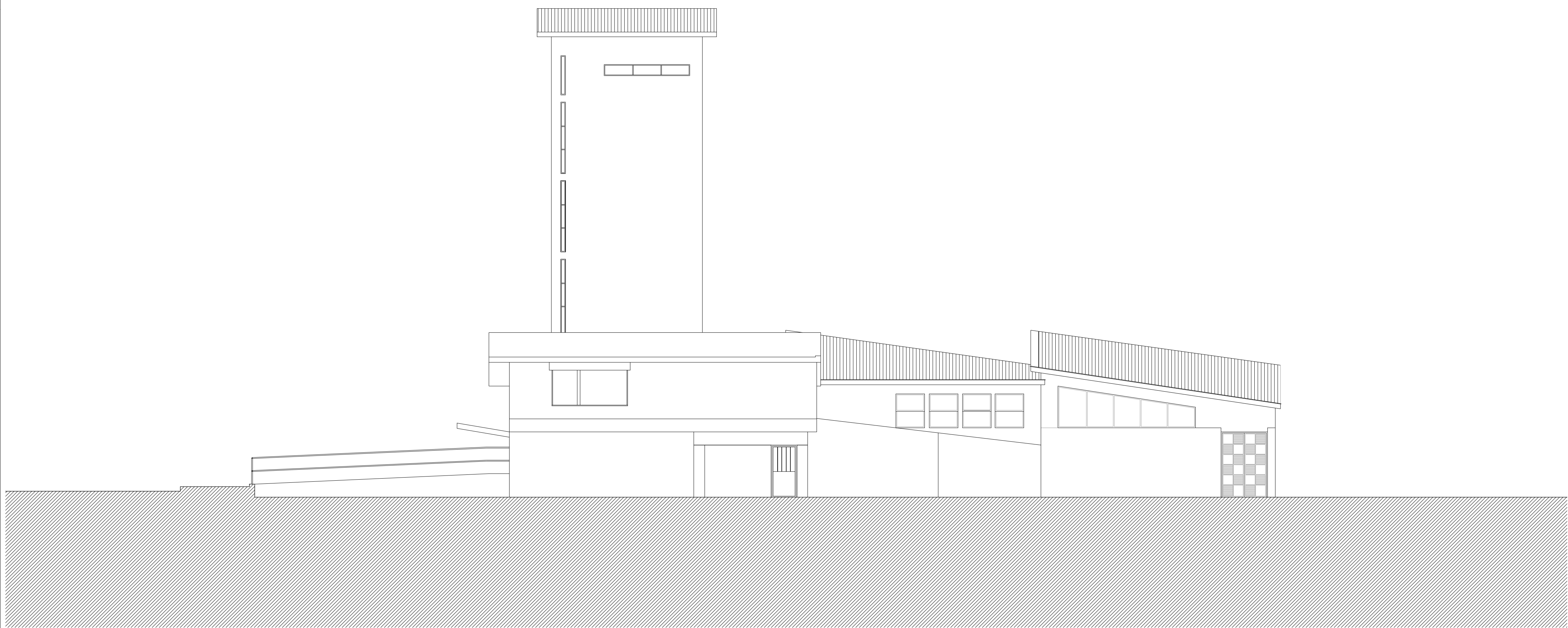
ALÇADO SUDOESTE
