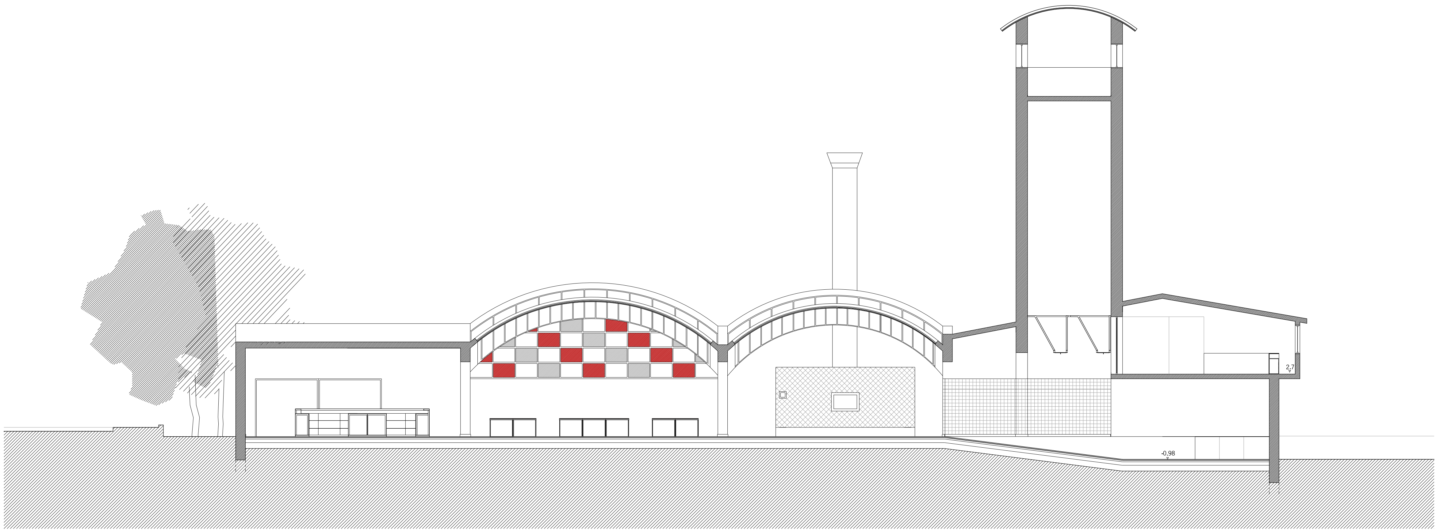
CORTE DD'
