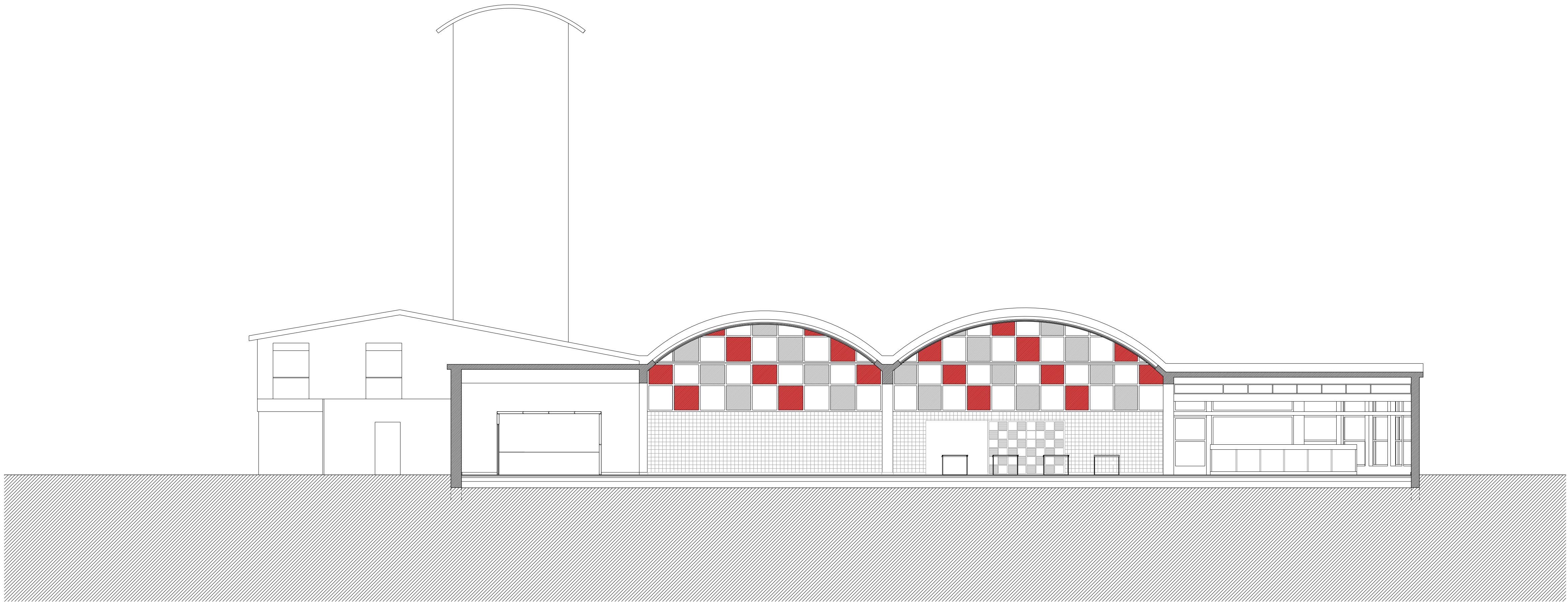
CORTE CC'
