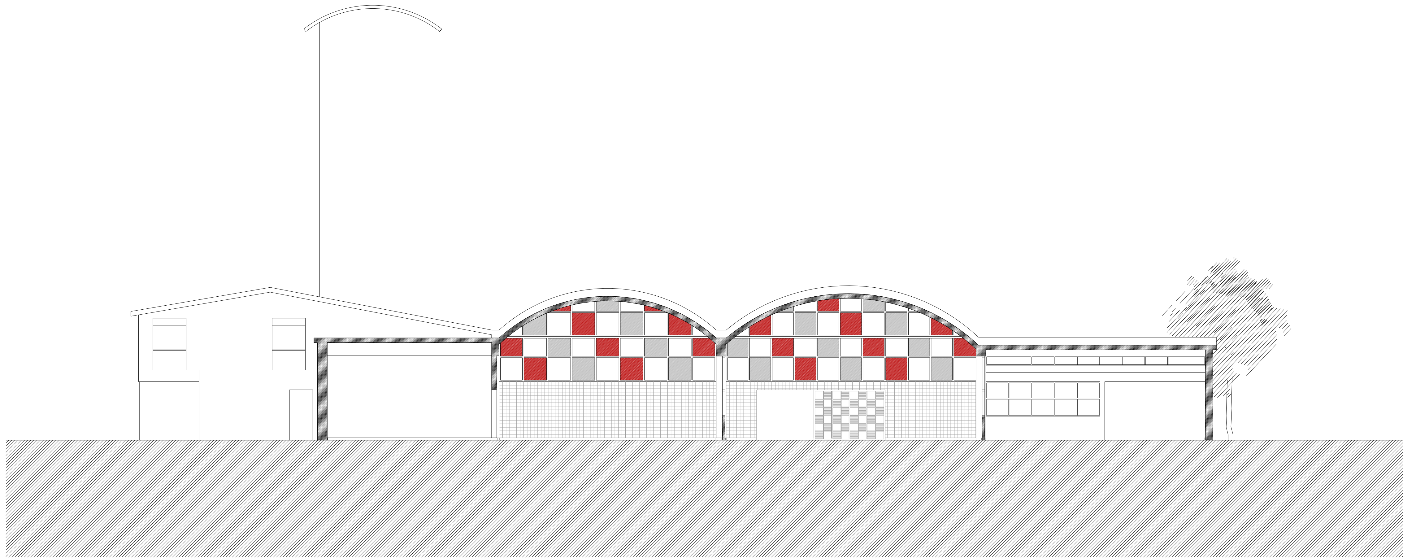
CORTE DD'
