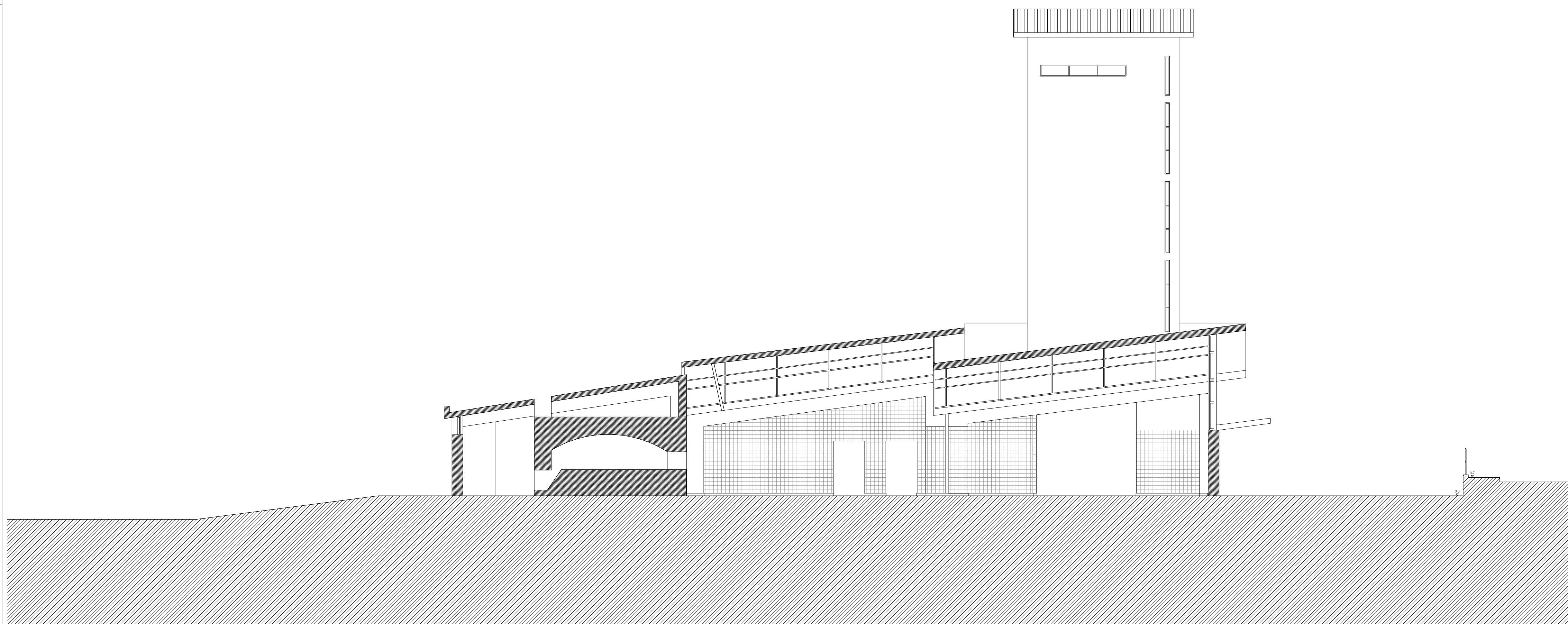
CORTE BB'
