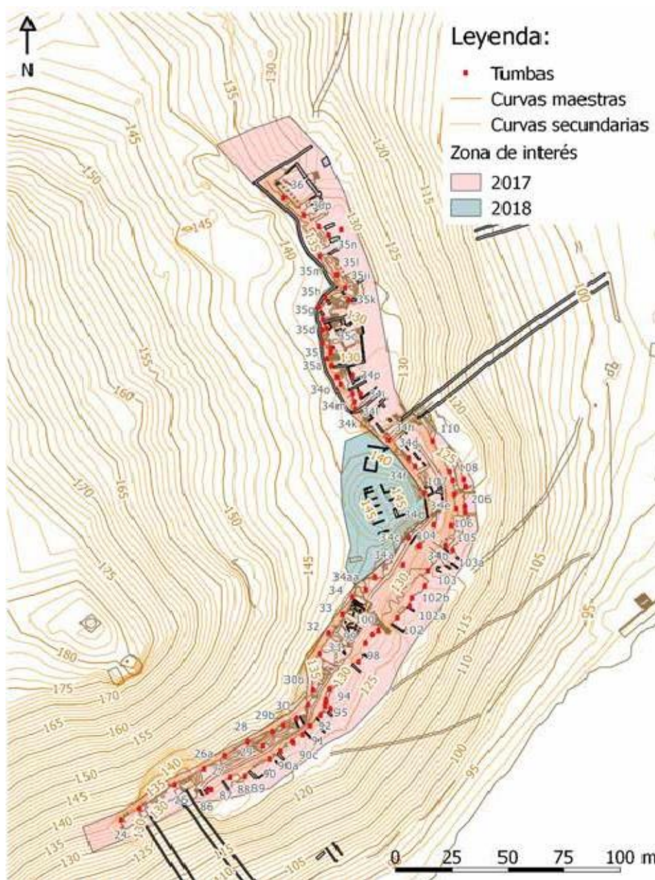
Figura 24. Levantamento topográfico com a localização de todos os Túmulos identificados até ao momento.
