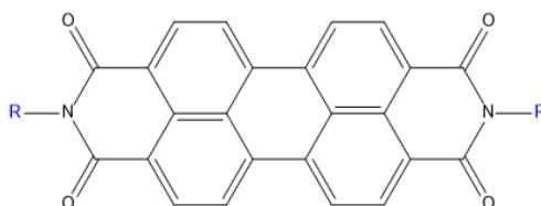
Figura 1: Estrutura química de uma molécula de perileno bismide modificada com um grupo R.
